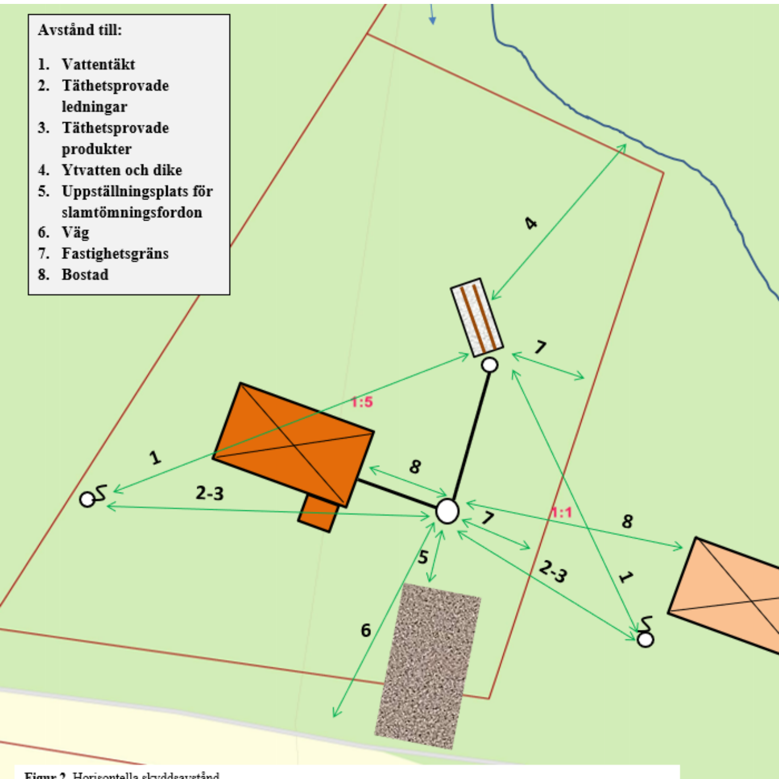
Figur 2. Horisontella skyddsavstånd
